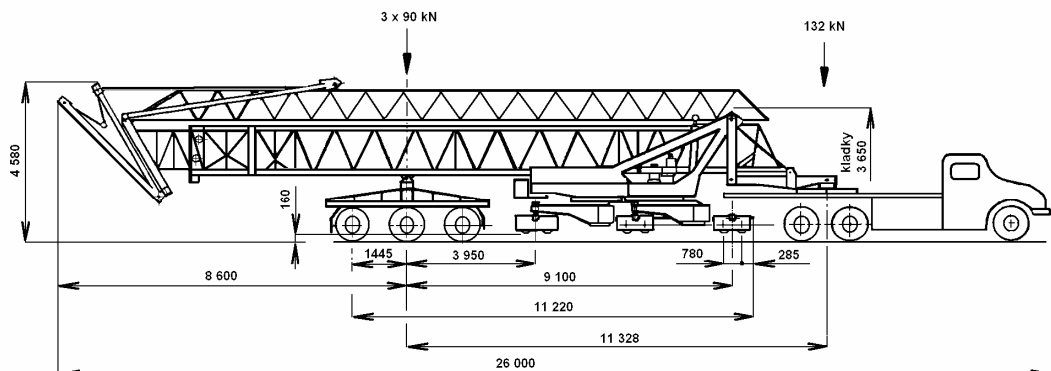
Přepravní poloha na podvozku a tahači
